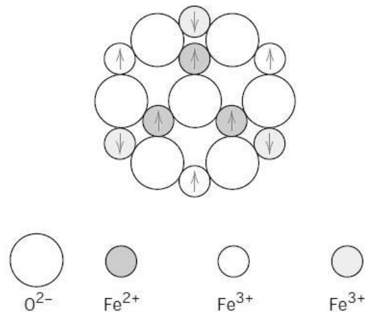
Slika 10: Prikaz magnetskih momenata kod ferimagneta Fe_3O_4 . [9]
