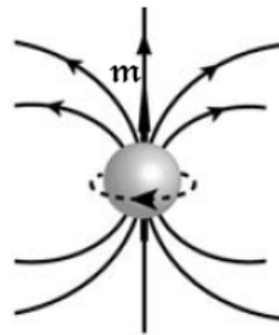
Slika 3: Magnetski moment povezan spinskim kutnim momentom elektrona [10]
