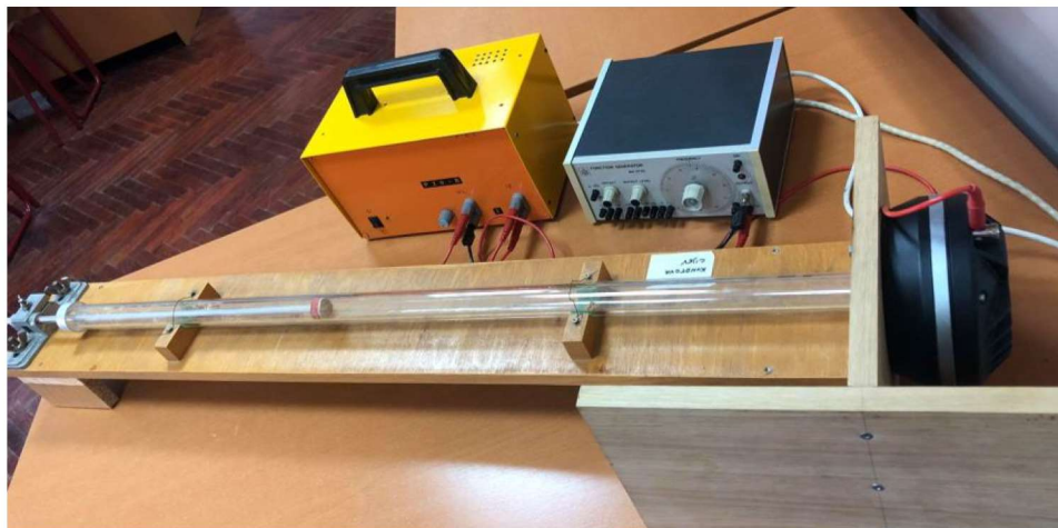
Slika 22. Eksperimentalni postav.
