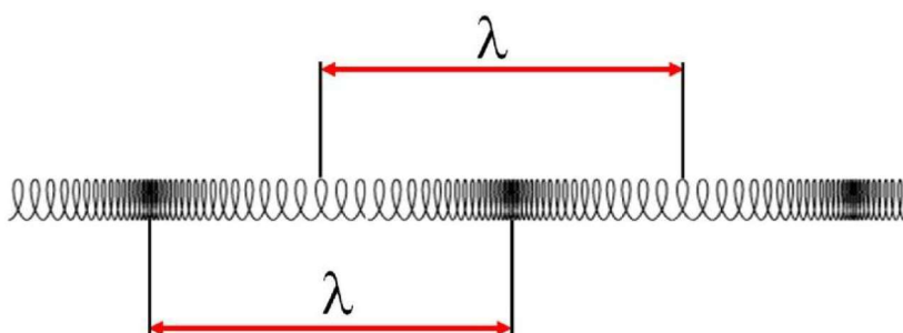
Slika 4. Longitudinalni val sastoji se od niza zgušnjenja i razrjeđenja. To su poremećaji koji putuju sredstvom i prenose energiju. Valna duljina longitudinalnog vala jednaka je razmaku između dvaju susjednih zgušnjenja, odnosno dvaju susjednih razrjeđenja [10].
