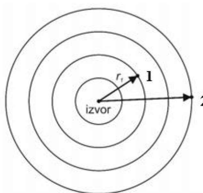
Slika 5. Intezitet zvuka opada s kvadratom udaljenosti od izvora [1].
