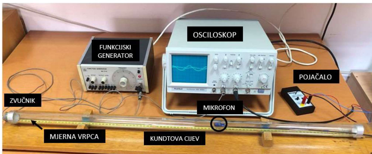
Slika 25. Eksperimentalni postav.
