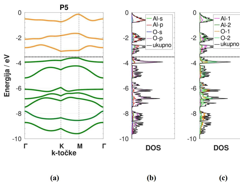
Slika 21. (a) Struktura elektronskih vrpca oksida aluminena koji nastaje kad se molekula kisika postavi u položaj P5. (b) Gustoća stanja elektrona atoma aluminija i atoma kisika u oksidu aluminena po orbitalama s i p koji nastaje kad se molekula kisika postavi u položaj P5. (c) Gustoća stanja elektrona atoma aluminija i atoma kisika oksida aluminena koji nastaje kad molekulu kisika postavimo u položaj P5. Horizontalna istočkana linija je fermijev nivo. Zelene vrpce su valentne vrpce, a narančaste su vodljive vrpce.
