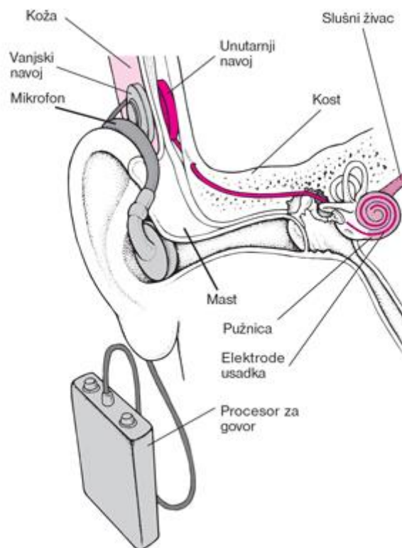
Slika 13. Umjetna pužnica [36]
