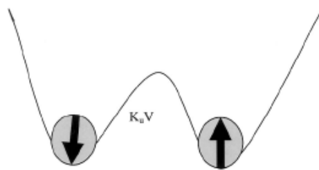
Slika 4. Dvostruka potencijalna jama s energijskom barijerom između.
