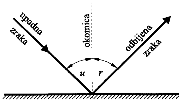
Slika 1. Refleksija svjetlosti na ravnom zrcalu [15]
