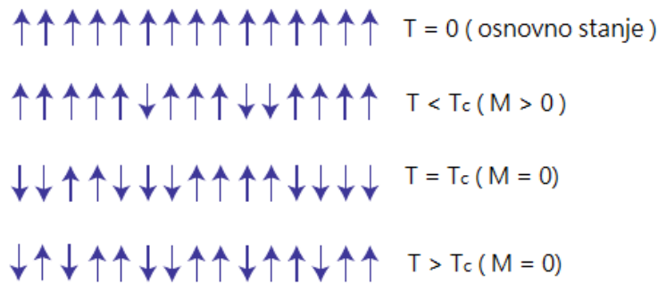
Slika 5: Spinsko uređenje. [1]
