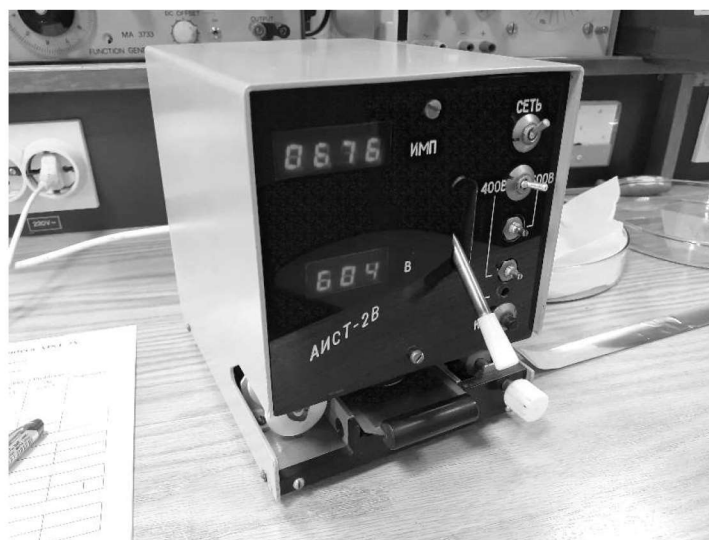
Slika 5.5.: Brojač iskri АИСТ-2В (ru. АИСТ-2В) korišten pri mjerjenju. Gornji ekran prikazuje broj mjerjenja, a donji napon kroz detektorski film. S desne strane prožet je Mylarov film koji se koristi za mjerjenje. Ručkom se prislanja elektroda na film.
