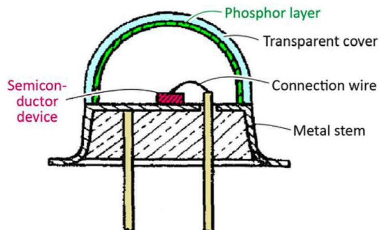
Slika 11. Poprečni presjek LED diode s fosfornim premazom [15]
