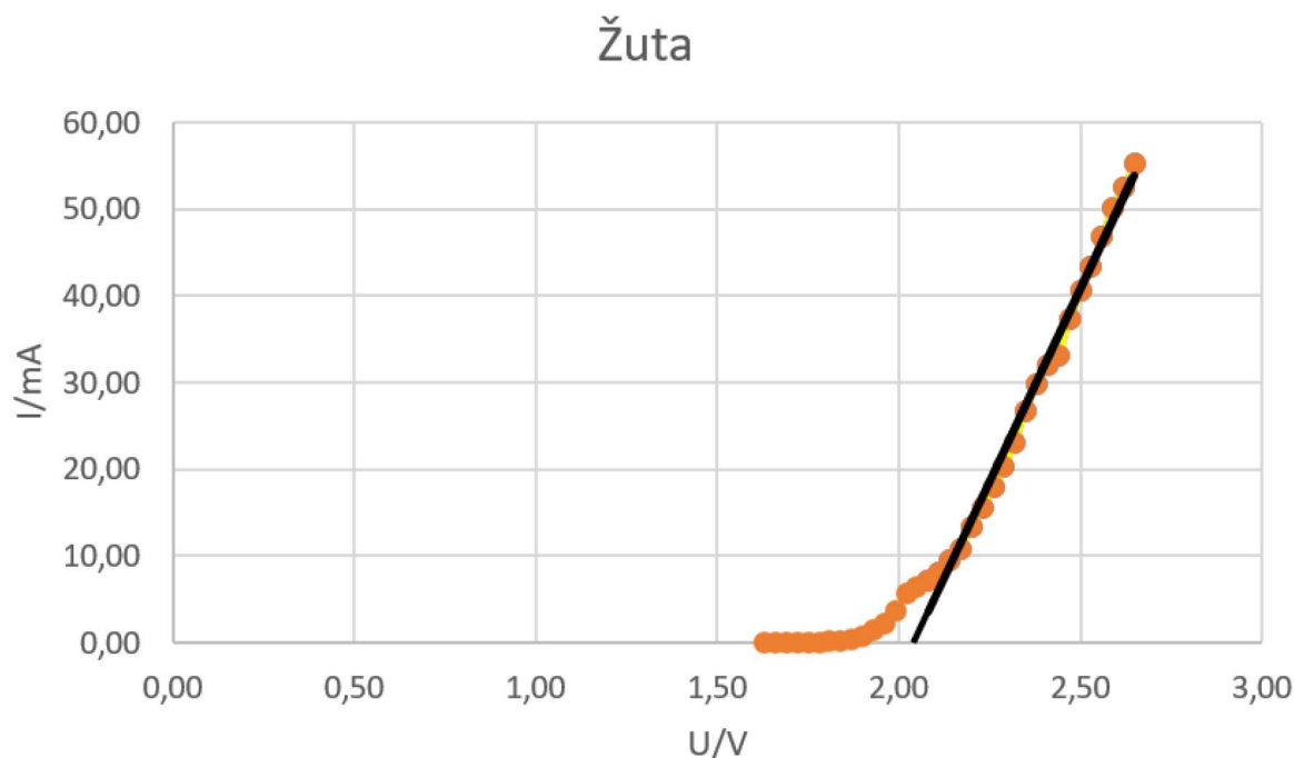
Graf 3. Strujno-naponska karakteristika žute LED diode
