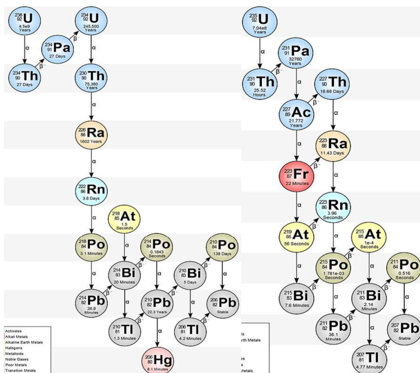
Slika 4. Lanci radioaktivnog raspada ^{238}\text{U} i ^{235}\text{U}
