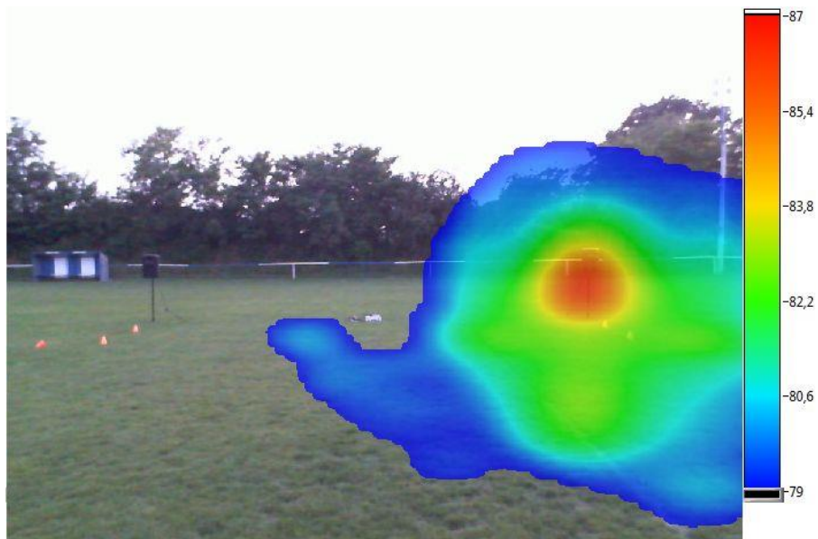
Slika 26. Akustička slika desnog zvučnika ( d=18,48 m).
