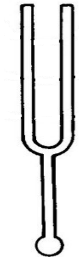
Slika 6. Glazbena vilica [13]
