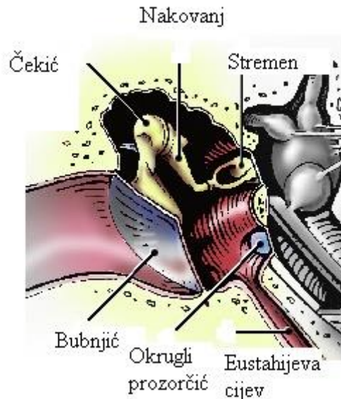
Slika 10. Srednje uho [2]
