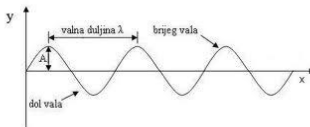
Slika 1. Sinusoidalni val [19]
