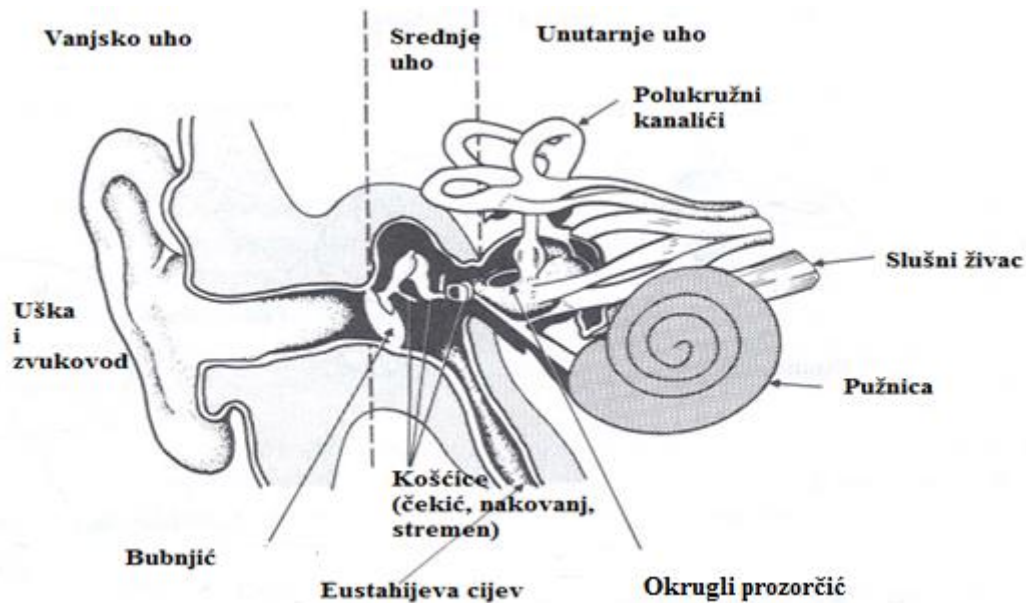
Slika 8. Uho [34]
