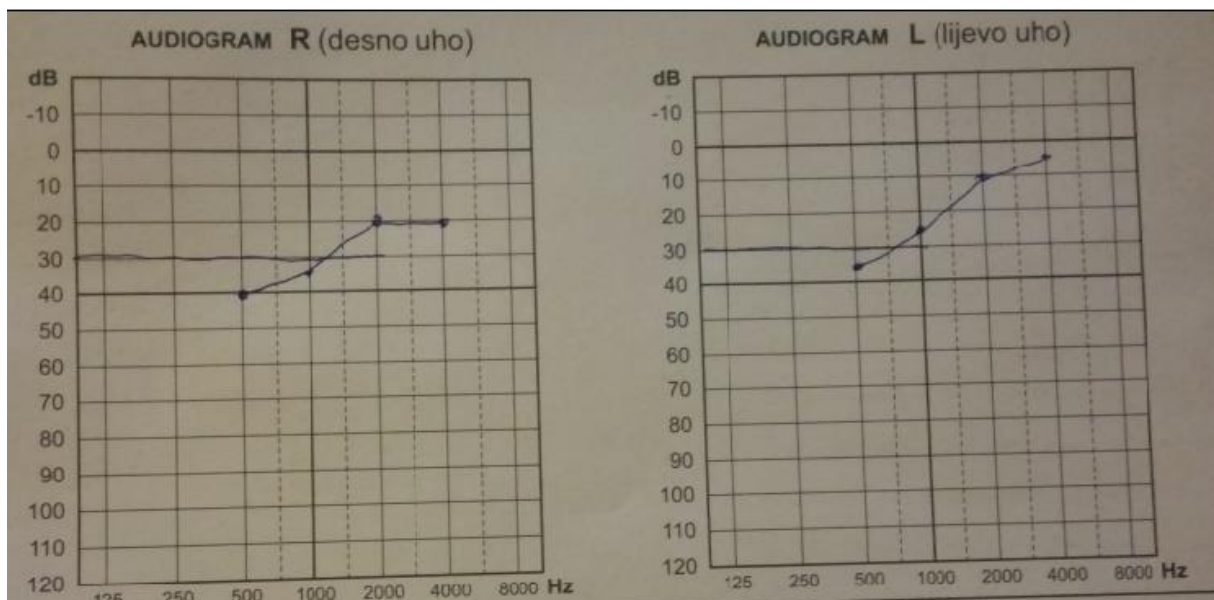
Slika 12. Audiogram [1]
