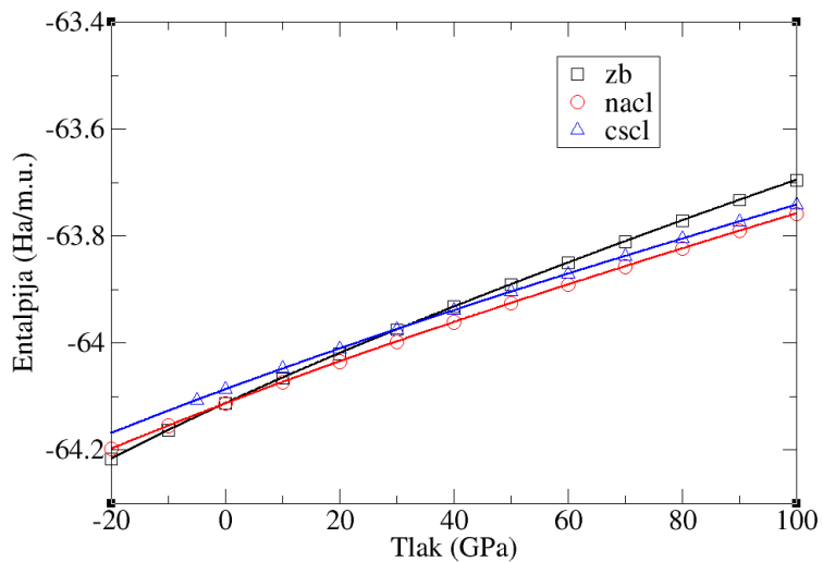
Slika 4.20: Prikaz grafa entalpije u ovisnosti o tlaku za CuN u različitim fazama.
