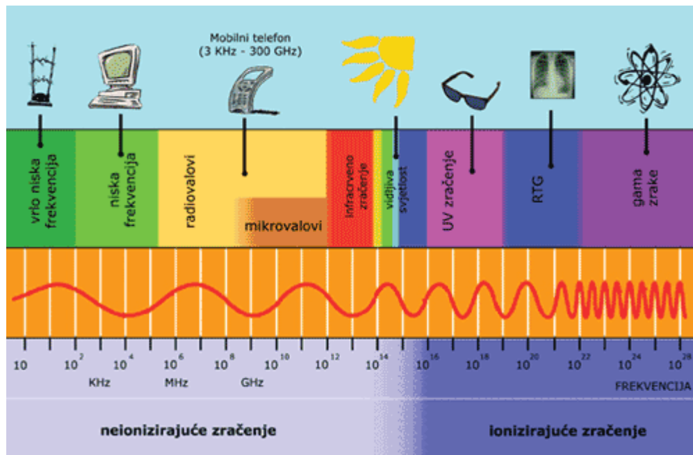
Slika 2. Spektar elektromagnetskog zračenja [1]
