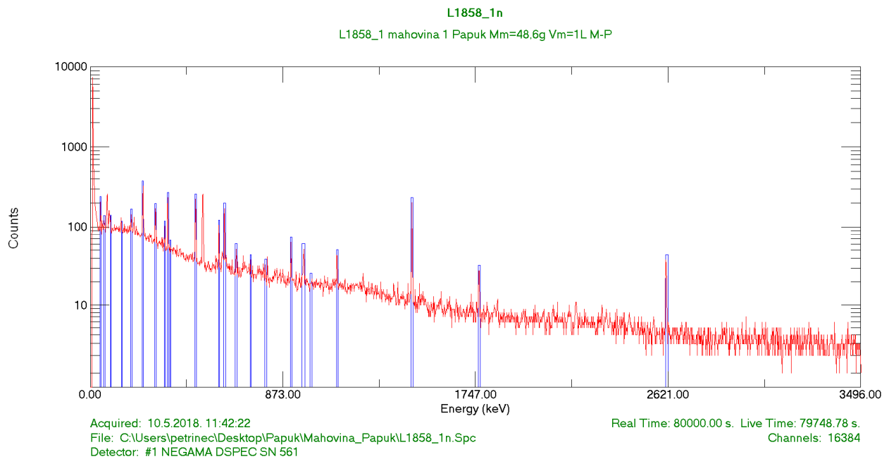
Slika 10. Spektar gama zračenja uzorka mahovine
