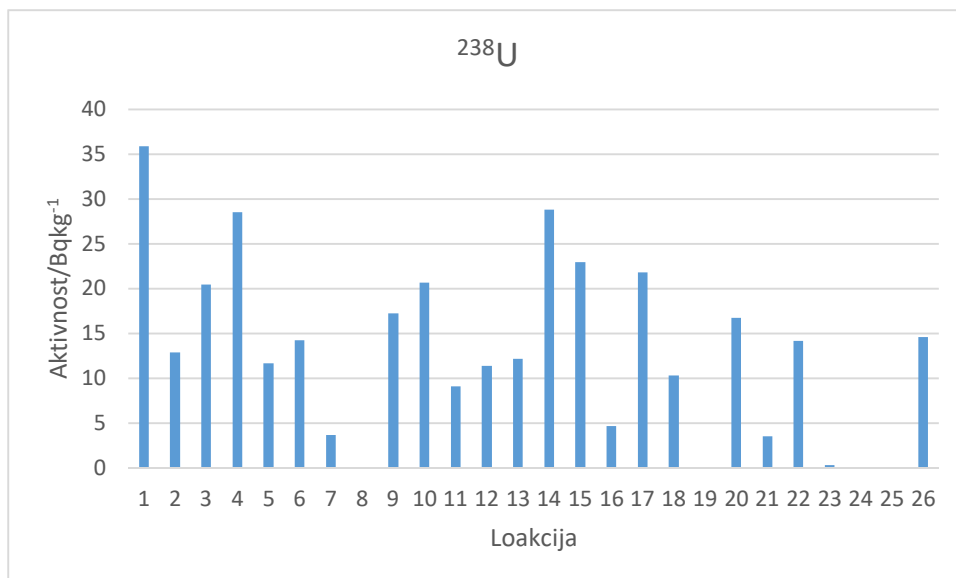
Grafikon 2. Koncentracija aktivnosti ^{238}\text{U}
