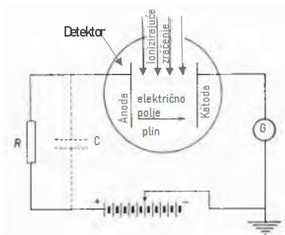
Slika 7. Shema plinskih detektora [13]
