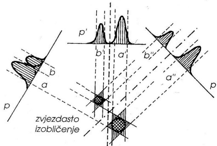
Slika 24. Zvjezdasto izobličenje. [2]
