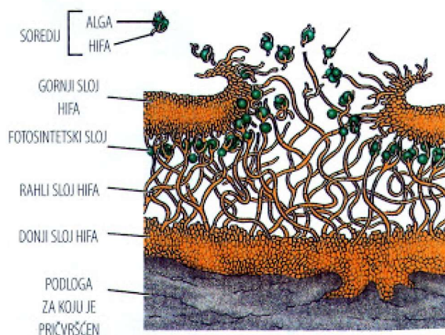
Slika 10. Građa lišaja. [27]
