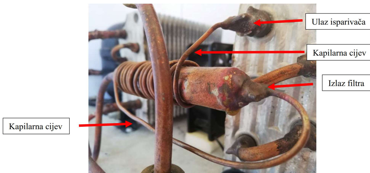
Slika 25. Povezivanje filtra i ulaza isparivača kapilarnom cijevi
