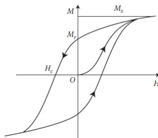
Slika 12: Krivulja histereze [13]
