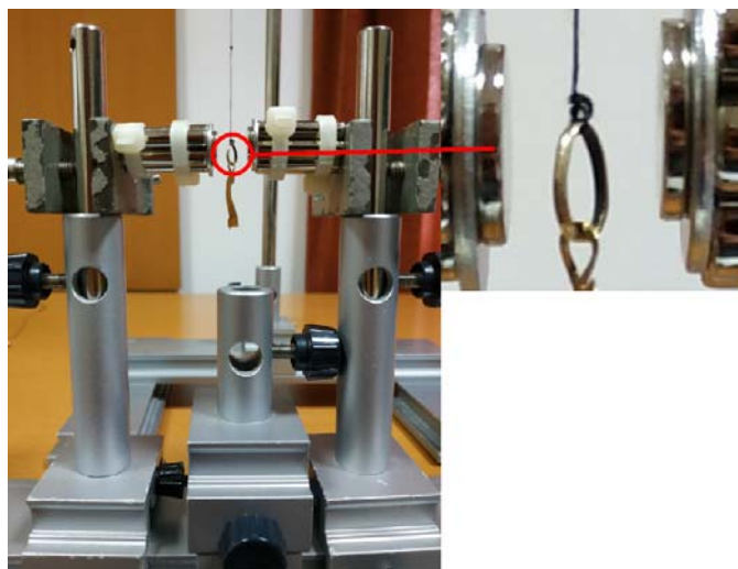
Slika 38: Ponašanje uzorka zlata u magnetskom polju
