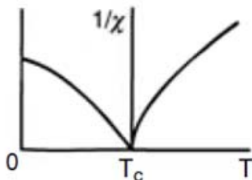
Slika 17: Ovisnost magnetske susceptibilnosti ferimagneta o temperaturi [9]
