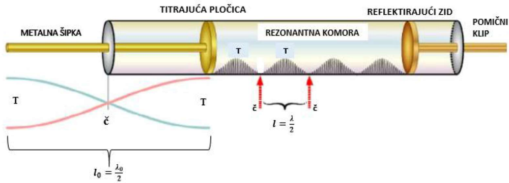
Slika 18. Shema pokusa, gdje Č predstavlja položaj čvora, a T položaj trbuha [20].
