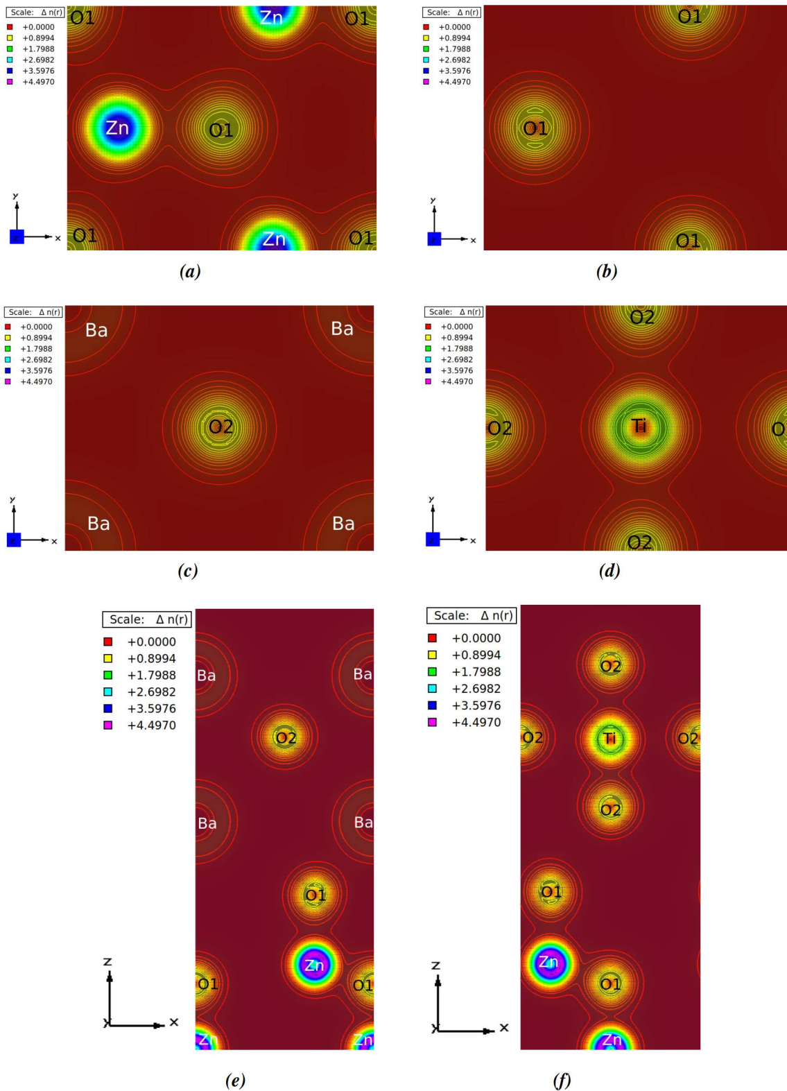
Slika 25: Ravninski prikaz gustoće naboja oko atoma. Slika (a) prikazuje gustoću naboja oko atoma cinka i kisika za plohu koja se nalazi na središtu između obje vrste atoma, slika (b) prikazuje gustoću naboja oko atoma kisika uz spoj struktura, (c) prikazuje gustoću naboja oko barija i kisika u BaO sloju, (d) prikazuje gustoću naboja u TiO 2 sloju. Ravnine prikaza, kao i vrijednosti gustoća za pojedinu boju prikazane su uz svaku sliku. Slike (e) i (f) obuhvaćaju atome obje strukture, odnosno gustoće oko atoma objaju strukture. Oznakom O1 označeni su atomi kisika ZnO strukture, dok su oznakom O2 označeni atomi kisika BaTiO 3 strukture.
