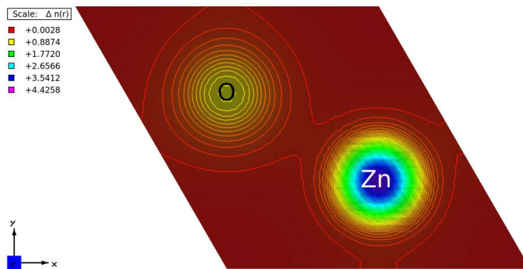
Slika 22: Ravinski prikaz gustoće naboja u x-y ravnini. Prikazana je ploha koja se nalazi na središtu između atoma kisika i cinka.
