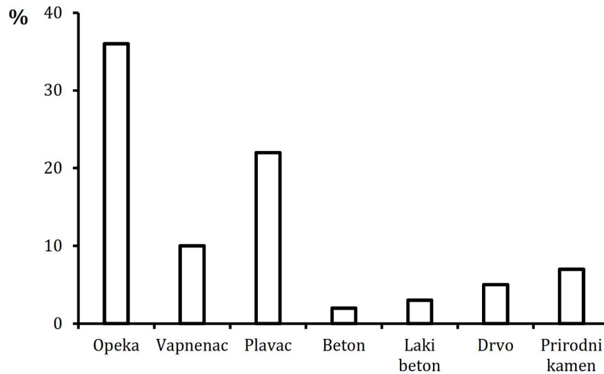
Slika 3.1.: Relativan broj stambenih zgrada s razinama radona koje prelaze 100 \text{ Bq m}^{-3} za različite građevinske materijale u Njemačkoj (Heller & Poulheim, 1992.).
