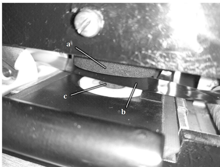
Slika 5.6.: Gornja elektroda (a) ručkom vidljivoj na slici 5.5. prislanja se preko Mylarova filma (b) na detektorski film (c) i tako s dnom brojača ispod čini kondenzator. Primjenom istosmjerne struje regulirane RC spojem, rupice u detektorskom filmu čine kratak spoj između elektroda tog kondenzatora, čime dolazi do preskoka, odnosno iskrenja koje brojač bilježi.
