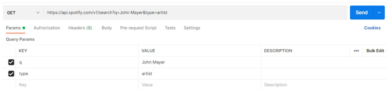
Slika 4.7 – Parametri GET zahtjeva s parovima ključ/vrijednost
