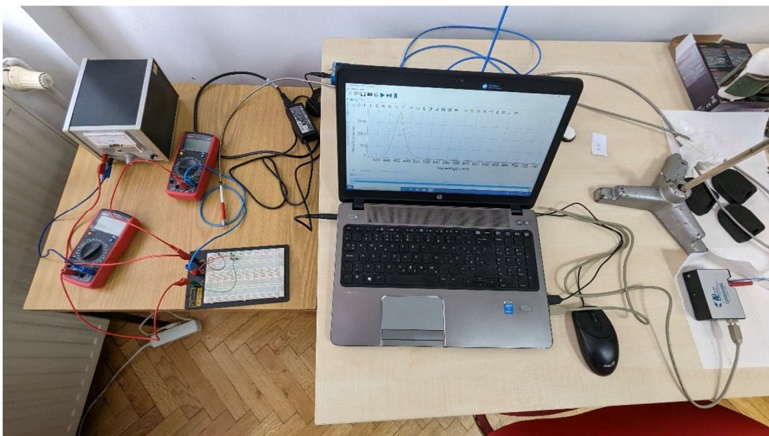
Slika 21. Eksperimentalni postava za određivanje valne duljine pomoću spektrometra
