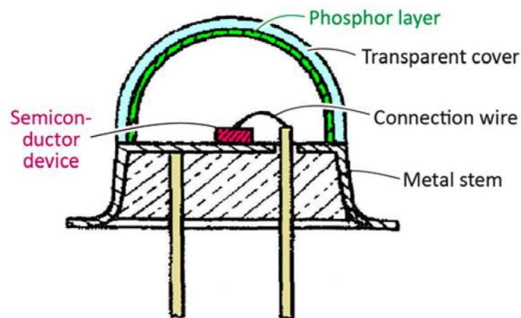
Slika 11. Poprečni presjek LED diode s fosforim premazom [15]
