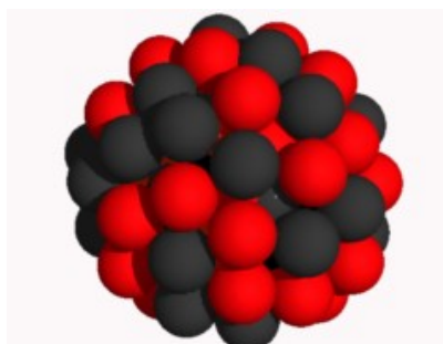
Slika 2 - Model atoma
