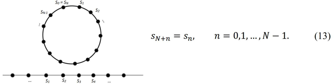
Slika 4: Slobodni i periodični rubni uvjeti 1D Isingova modela [vlastita izrada]
