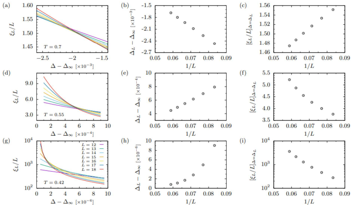
Slika 7: Analiza scalinga konačne dužine za korelacijsku dužinu [11]
