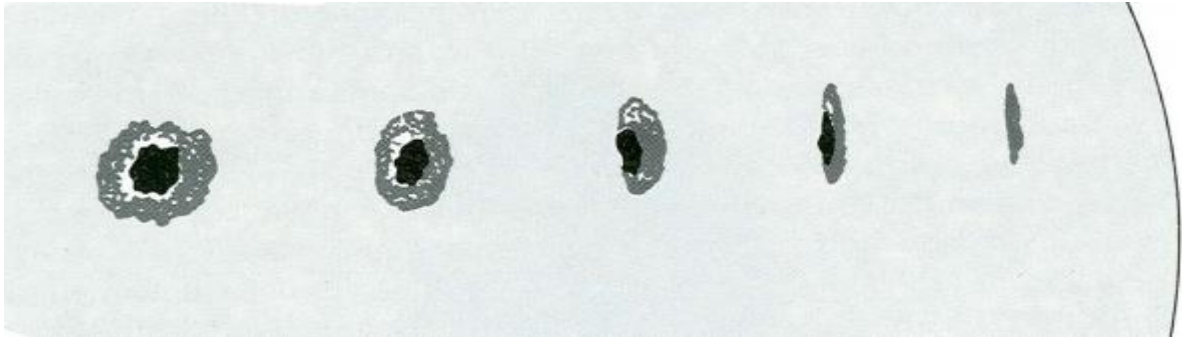
Slika 6. Wilsonov efekt [3]
