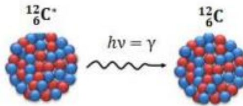
Slika 11: Gama raspad ugljika
