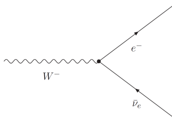
Slika 7: Feynmanov dijagram: Raspad W- bozona
