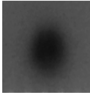
Slika 32: Film ozračen sedam dana ^{22}\text{Na}
