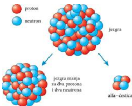
Slika 6: Alfa raspad radija
