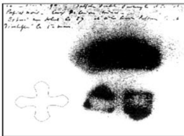
Slika 3: Prikaz radioaktivnih elemenata na fotografskoj ploči
