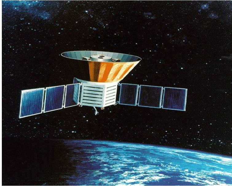
Slika 1: Izgled satelita COBE
