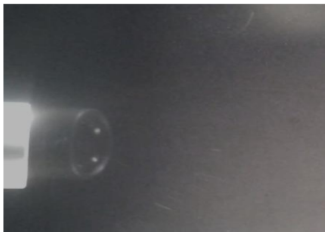
Slika 30. \alpha - zraka
