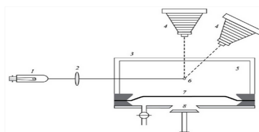
WILSONOVA KOMORA - 1. bjeskalica, 2. leća, 3. stakleno kućište, 4. fotoaparat, 5. prostor komore, 6. kondenzacijska jezgra, 7. pokretna membrana, 8. klip
