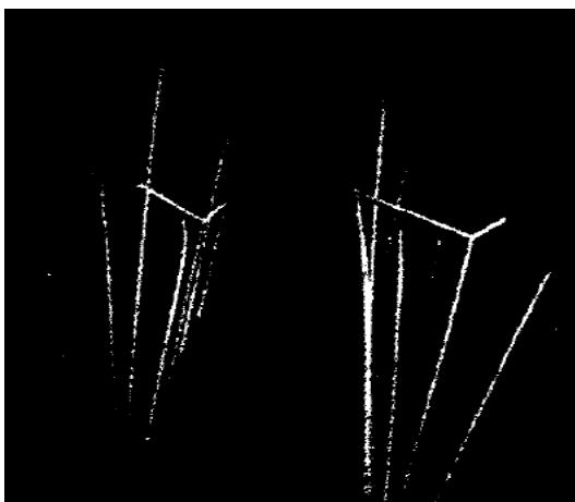
Slika 18. Elastični sudar alfa čestice s jezgrom kisika
