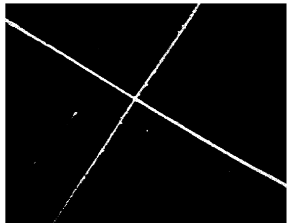
Slika 16. Razdvajanje iona (2)
