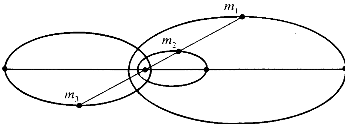
Slika 3. Eulerovo kolinearano rješenje za mase omjera m_1:m_2:m_3 = 1:2:3
