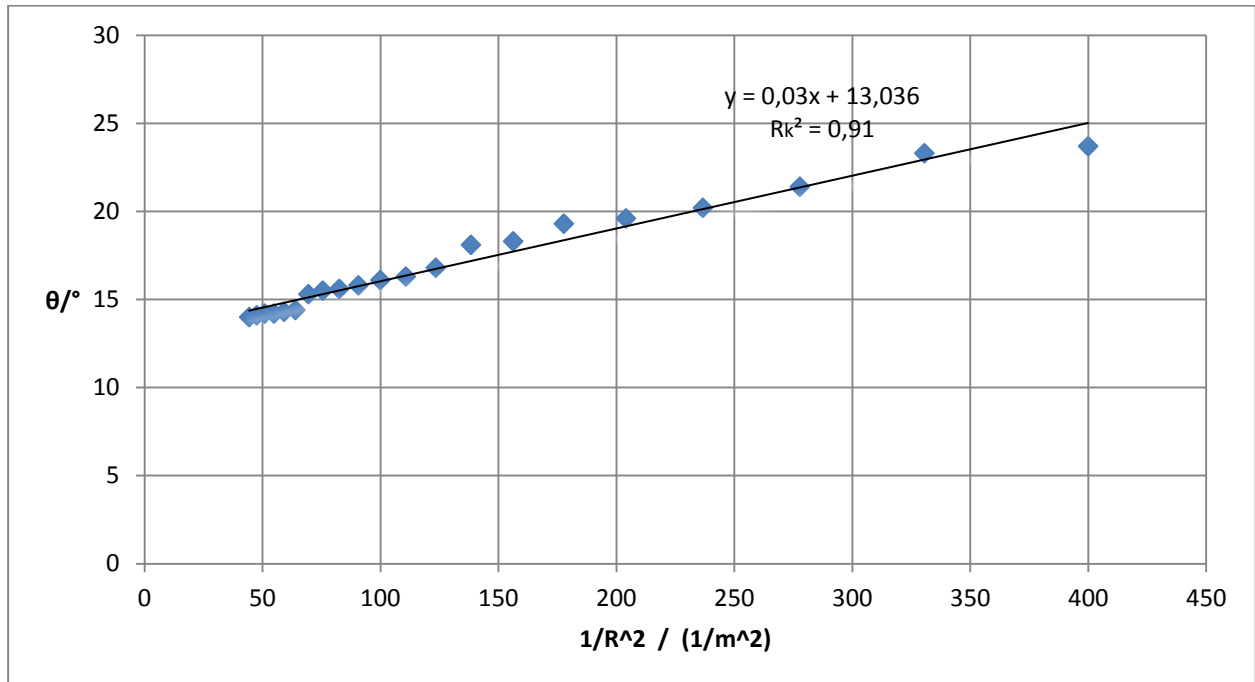
Graf 1: Ovisnost kuta torzije o recipročnoj vrijednosti kvadrata udaljenosti (\theta - \frac{1}{R^2})
