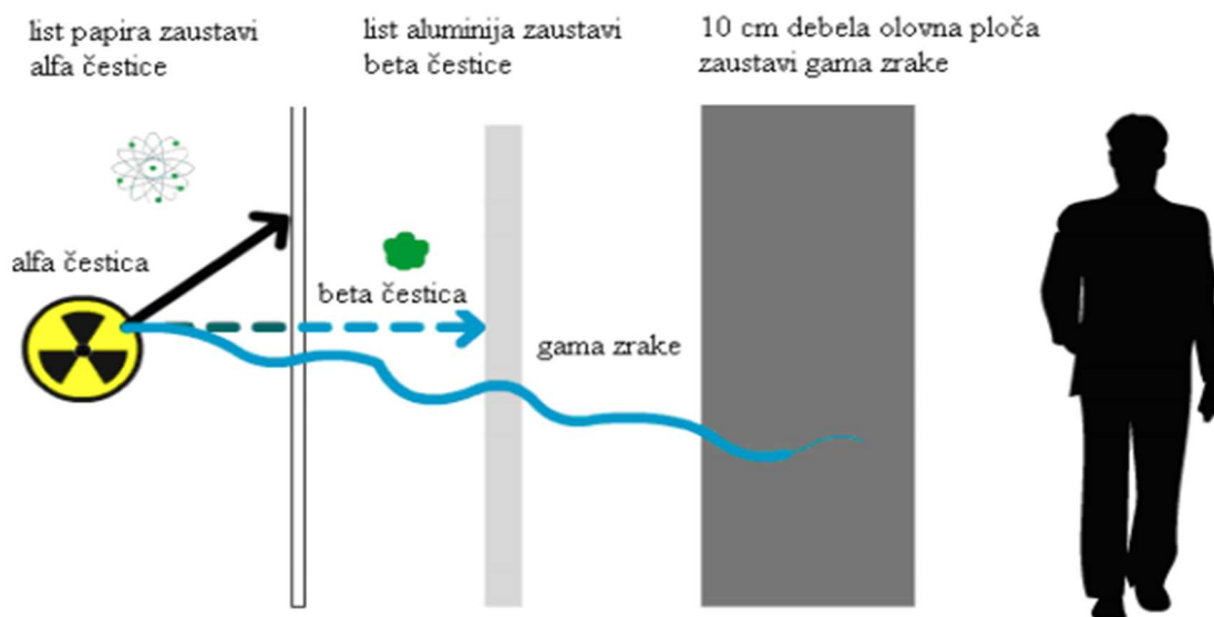
Slika 2. Prodornost alfa, beta i gama zračenja [4]
