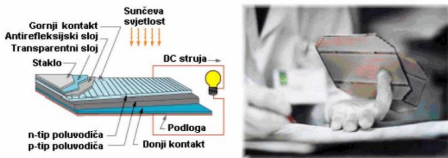
Slika 13. Solarna ćelija tankog filma [14]
