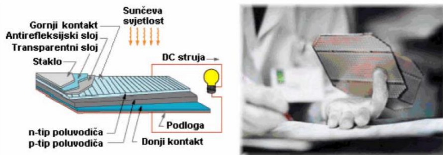
Slika 13. Solarne ćelija tankog filma [14]
