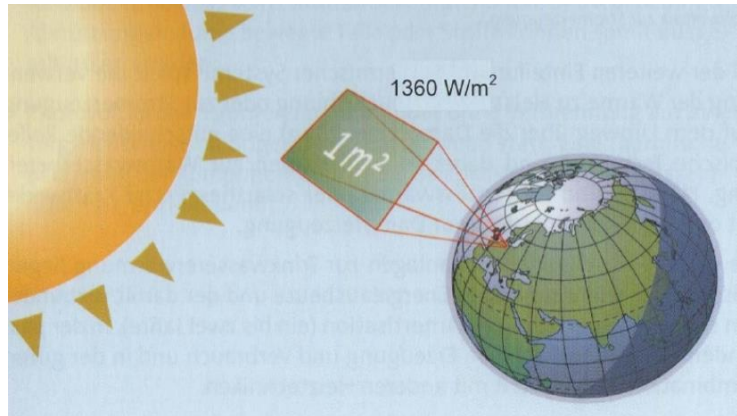
Slika 3. Solarna konstanta [13]
