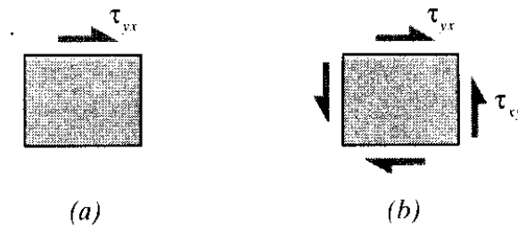
Slika 12. Posmična naprezanja na stranicu [25]
