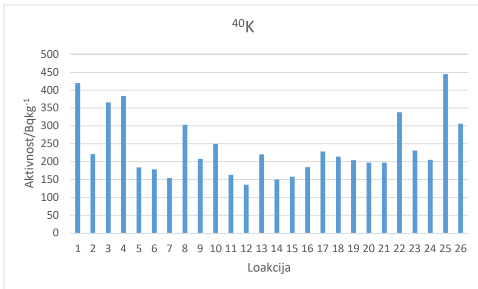
Grafikon 5. Koncentracija aktivnosti ^{40}\text{K}
